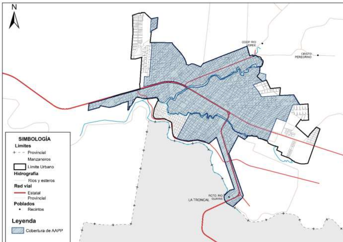
Mapa 68. Cobertura de agua potable
