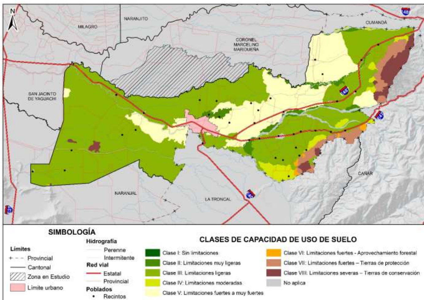
Mapa 12. Capacidad de Uso del Suelo
