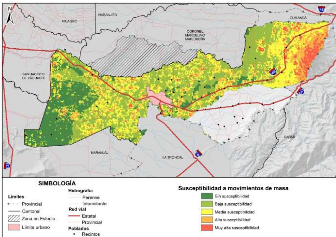
Mapa 14. Movimientos de masa
