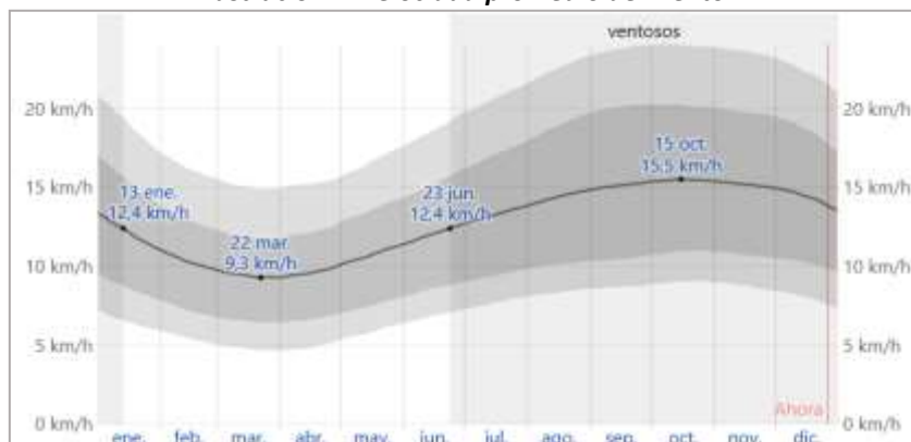
Ilustración 2. Velocidad promedio del viento
