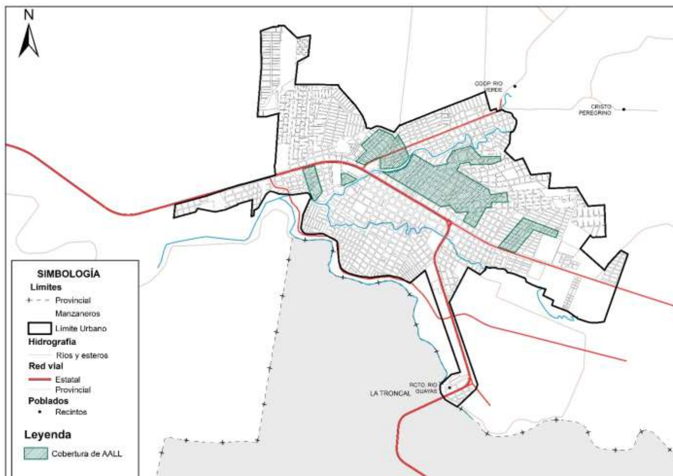
Mapa 74. Cobertura de alcantarillado pluvial
