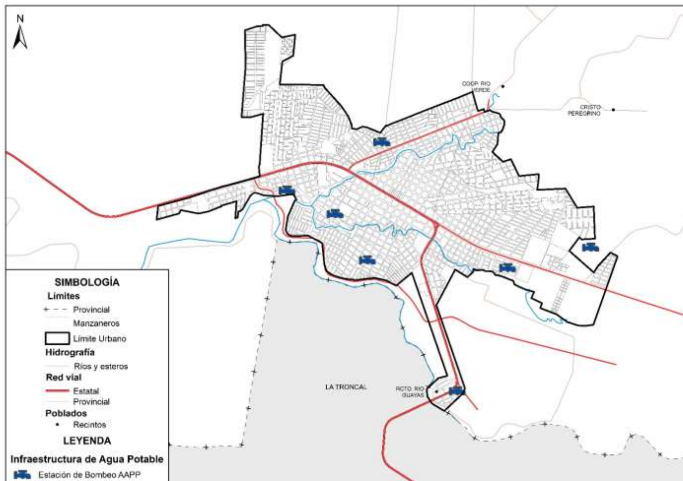
Mapa 71. Mapa de Estación de Bombeo
